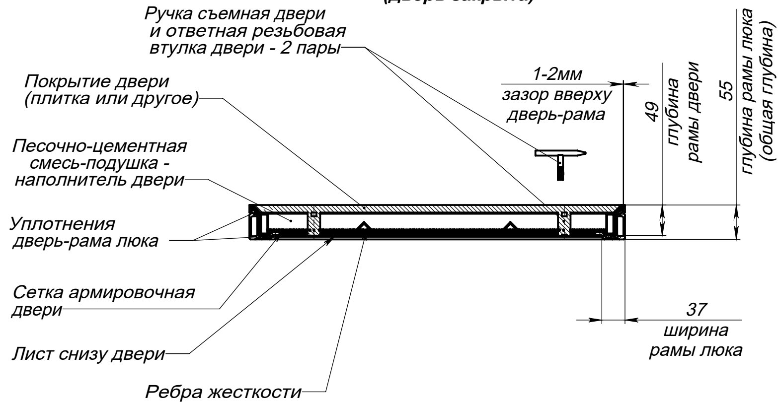
Вид сбоку на люк - в разрезе (дверь закрыта)
