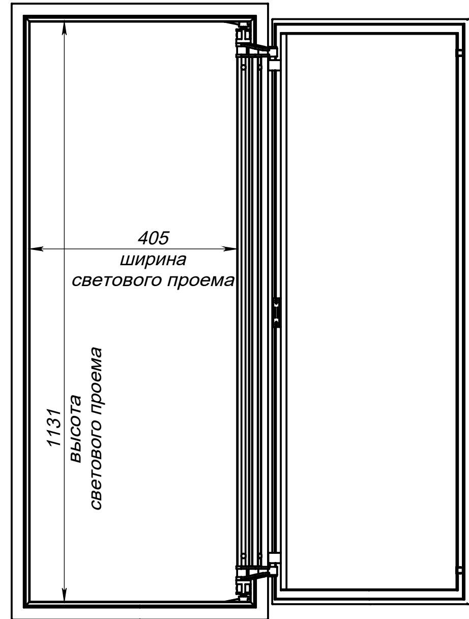
Вид спереди на люк (дверь открывается до 135 градусов)
