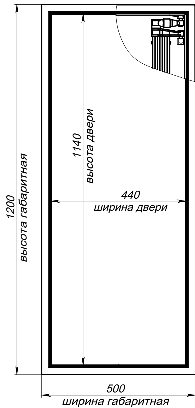
Вид спереди на люк (дверь закрыта)
