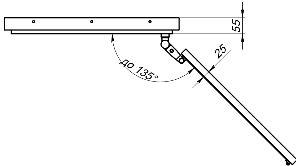
Вид сверху на люк (дверь открывается до 135 градусов)
