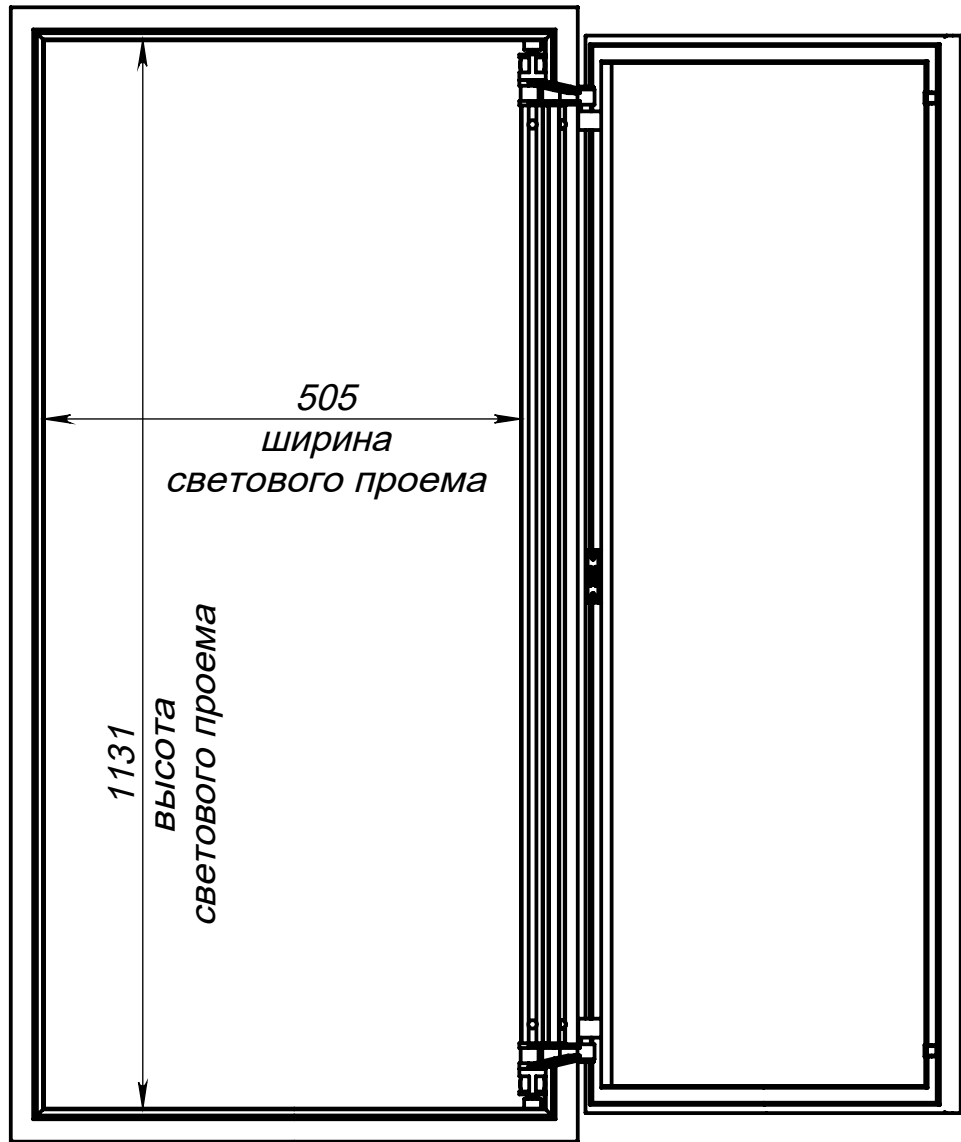
Вид спереди на люк (дверь открывается до 135 градусов)
