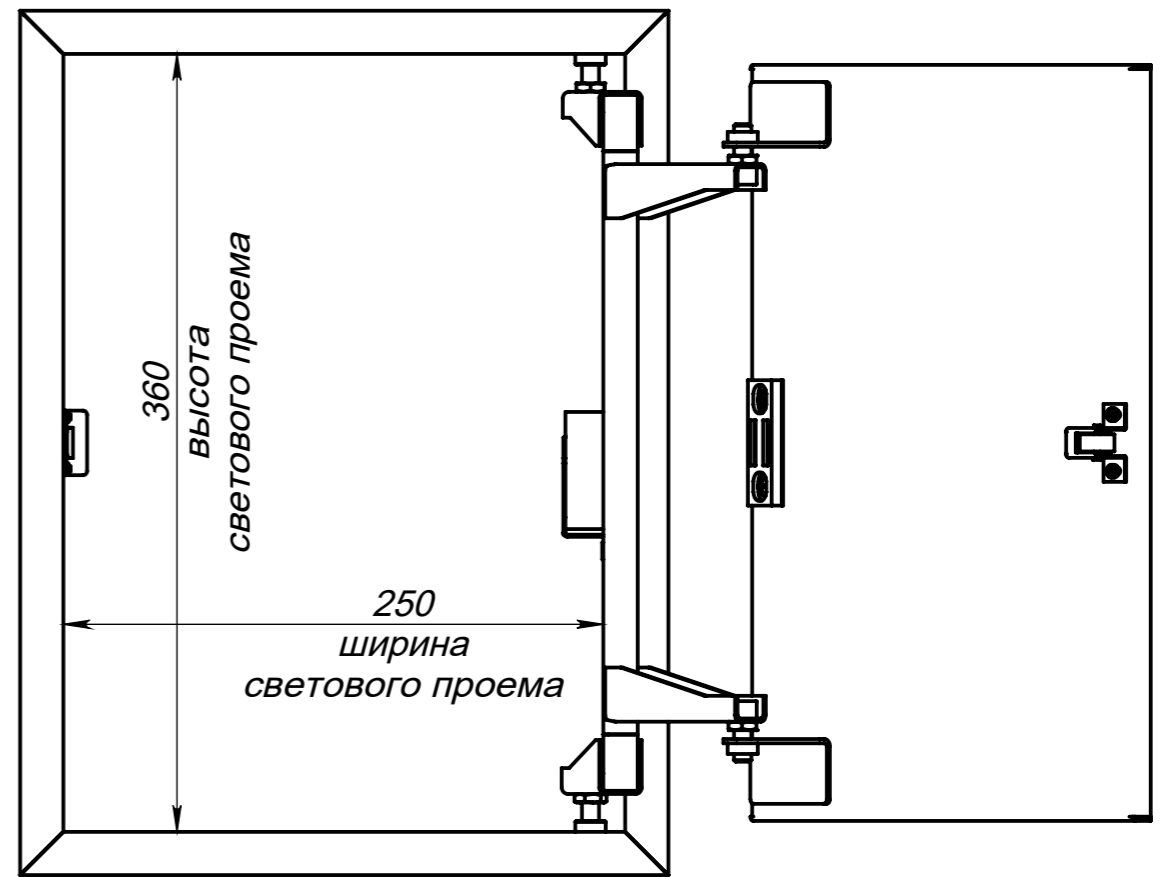
Вид спереди на люк (дверь открывается до 135 градусов)
