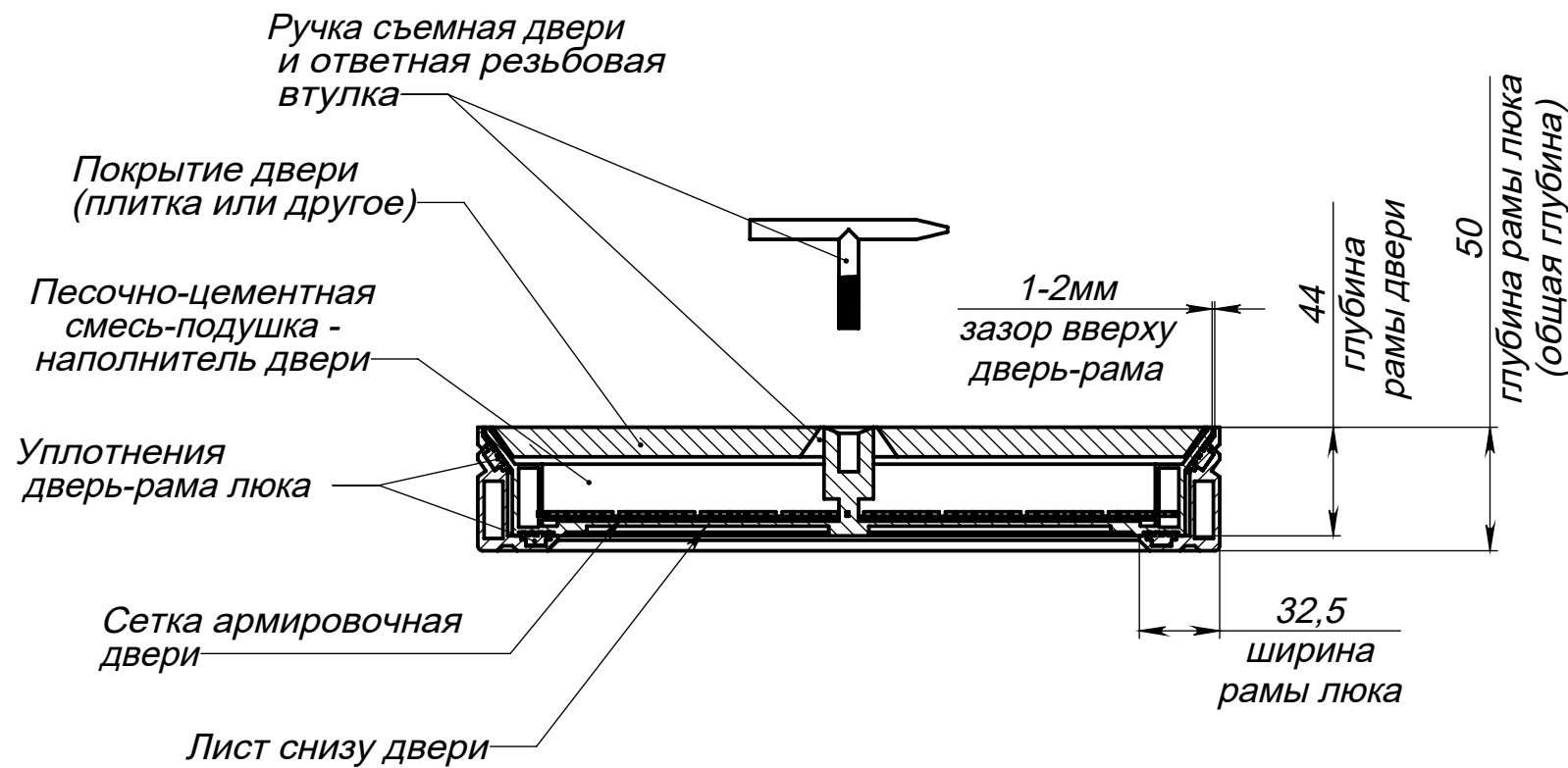
Вид сбоку на люк - в разрезе (дверь закрыта)
