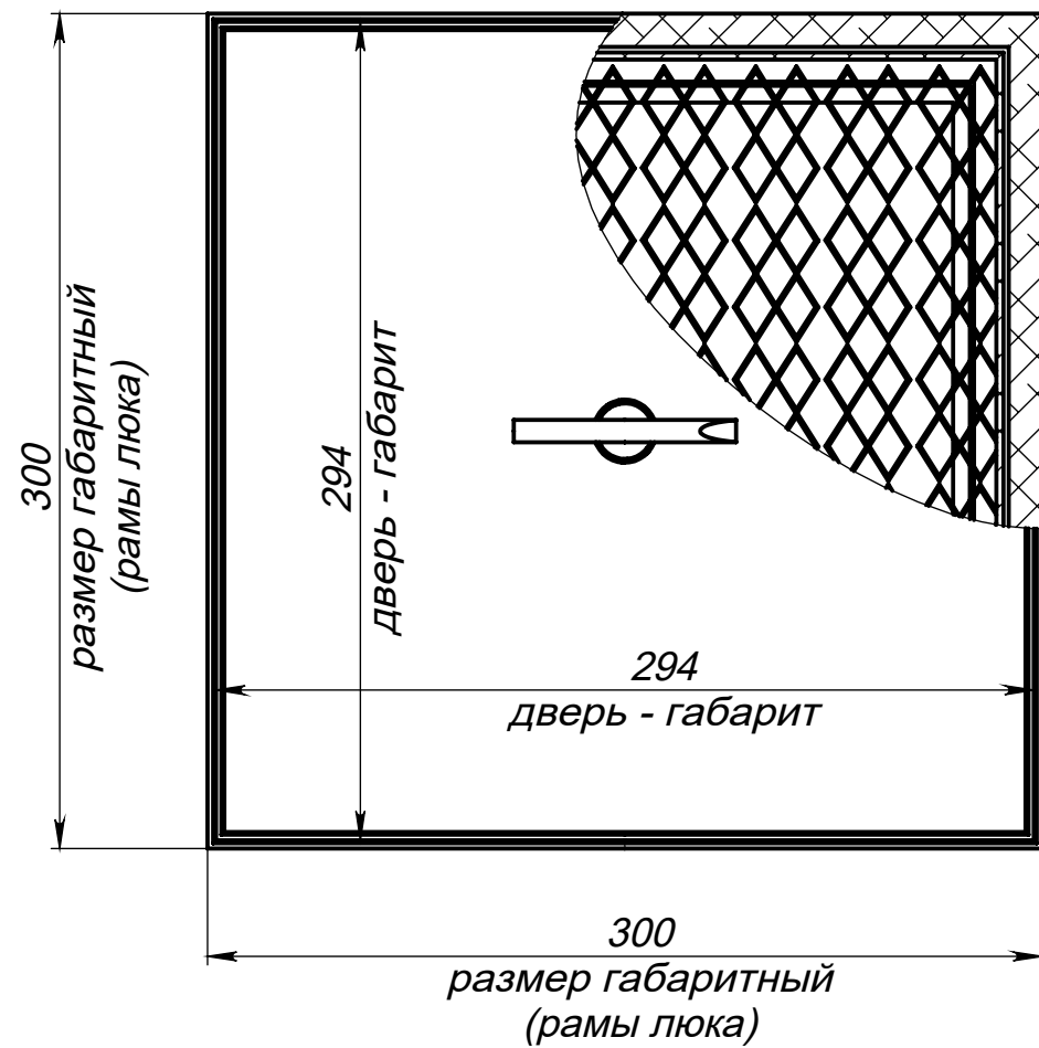
Вид сверху на люк (дверь со съемной ручкой)
