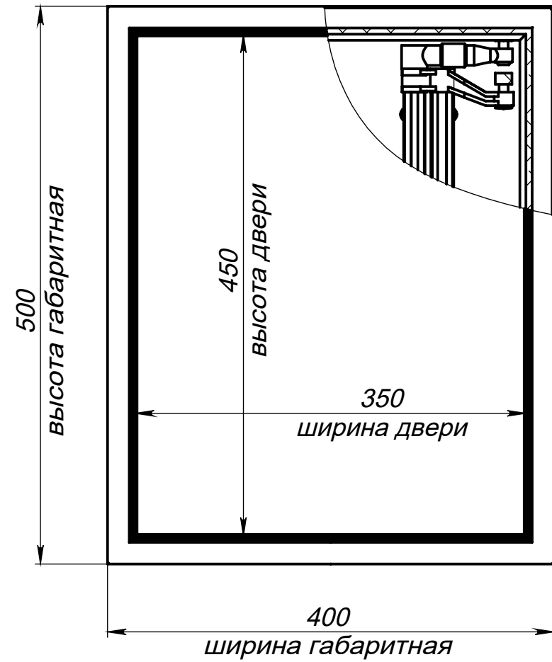
Вид спереди на люк (дверь закрыта)
