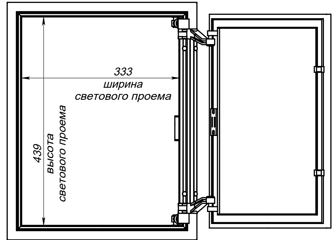
Вид спереди на люк (дверь открывается до 135 градусов)
