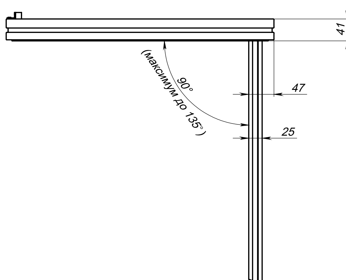
Вид сверху на люк (дверь открыта на 90 градусов)
