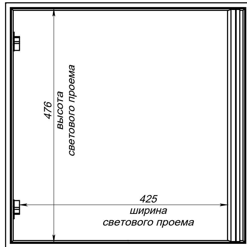
Вид спереди на люк (дверь открыта на 90 градусов)
