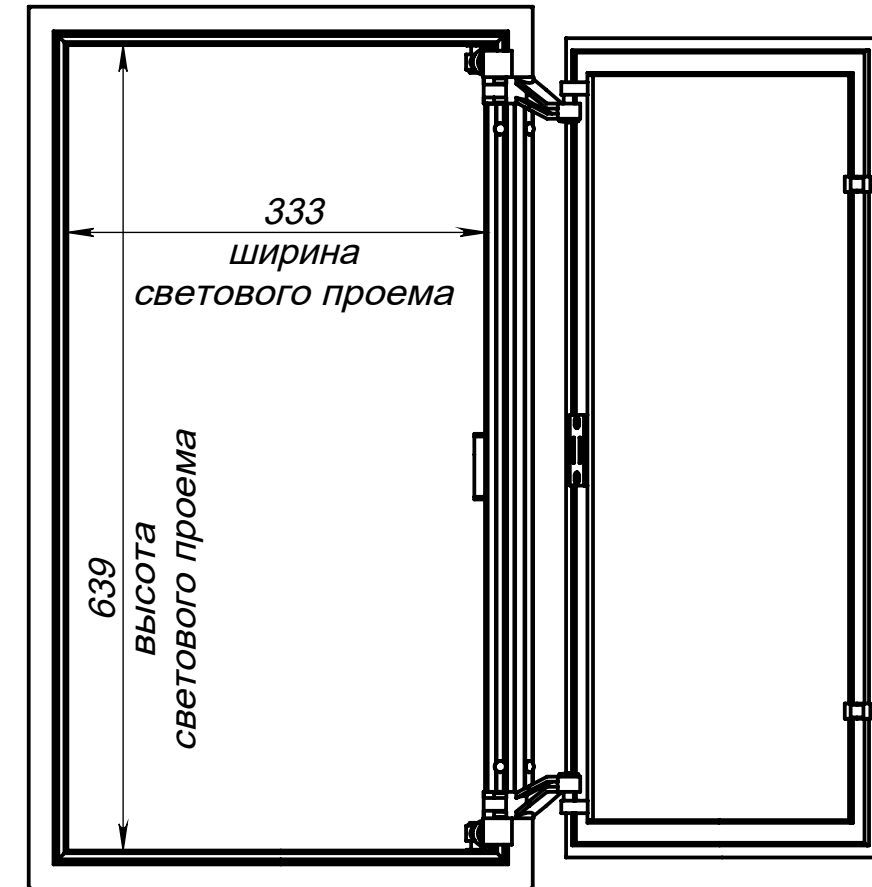
Вид спереди на люк (дверь открывается до 135 градусов)
