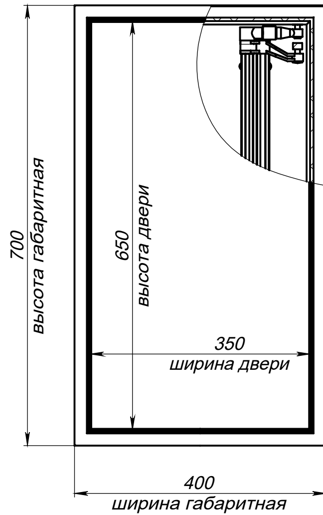
Вид сверху на люк - в разрезе (дверь закрыта)
