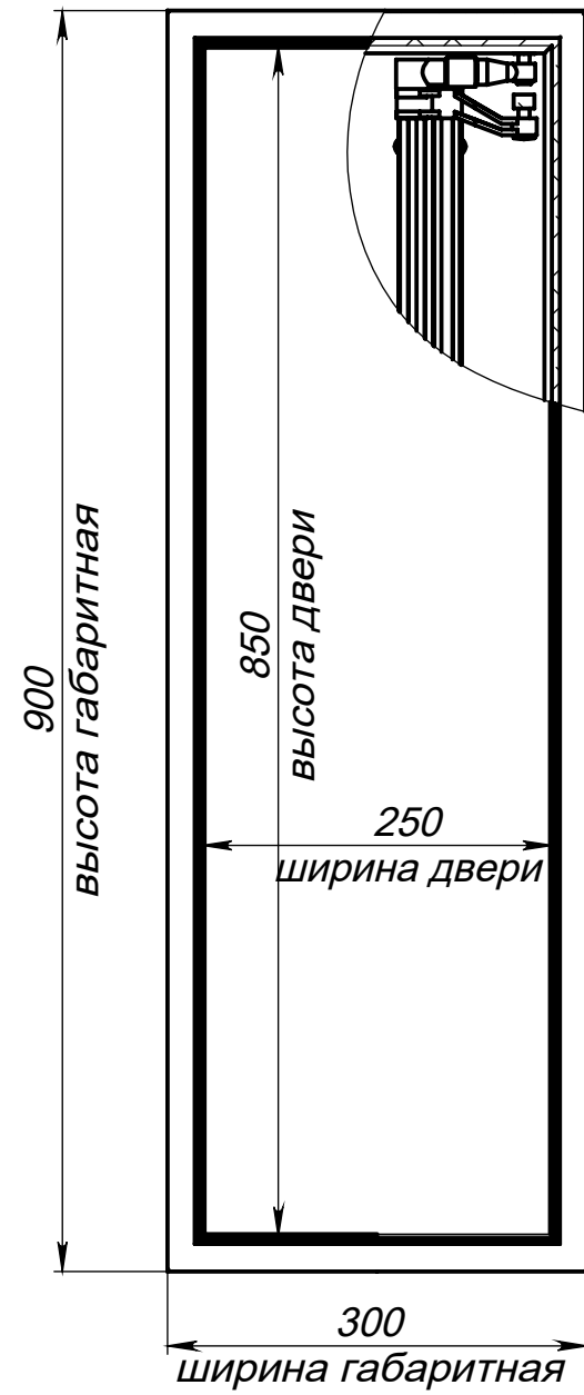
Вид спереди на люк (дверь закрыта)
