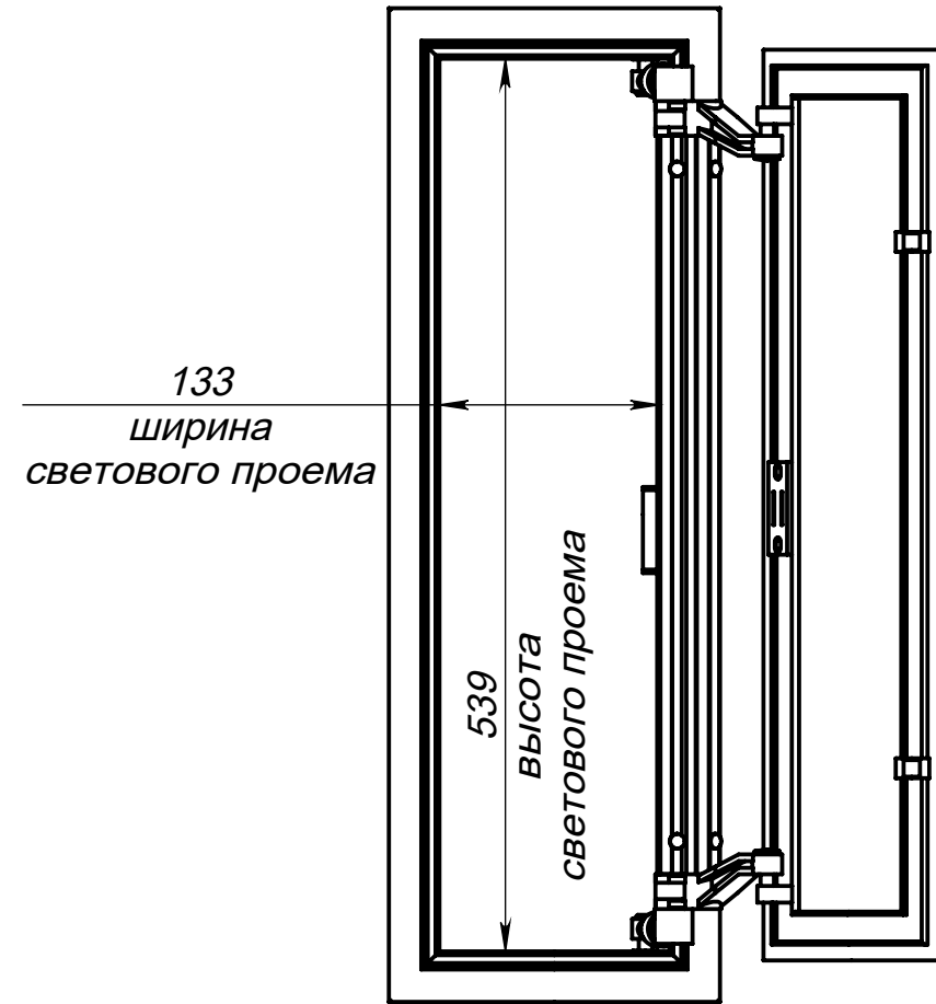
Вид спереди на люк (дверь открывается до 135 градусов)
