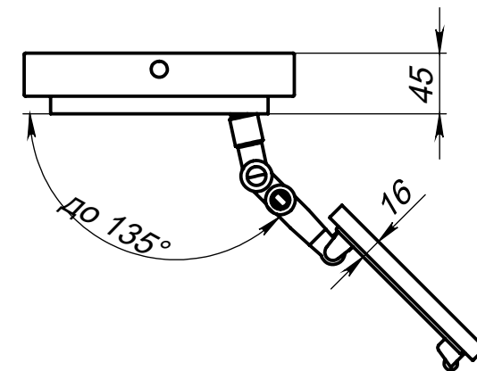
Вид сверху на люк (дверь открывается до 135 градусов)
