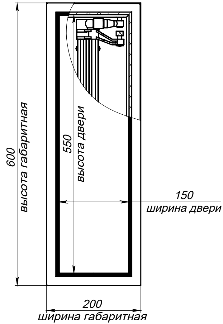
Вид спереди на люк (дверь закрыта)
