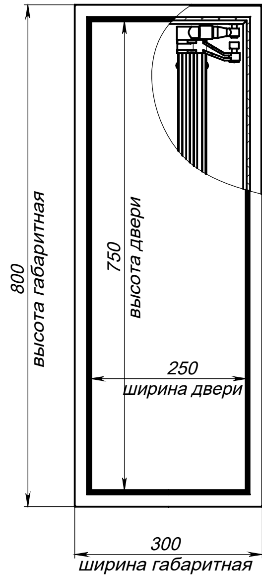
Вид спереди на люк (дверь закрыта)
