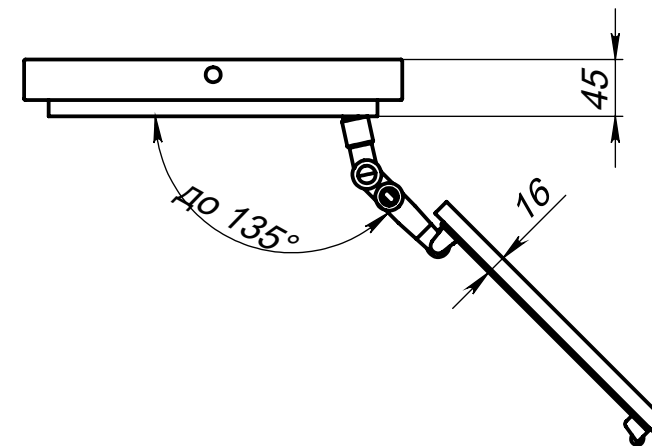
Вид сверху на люк (дверь открывается до 135 градусов)
