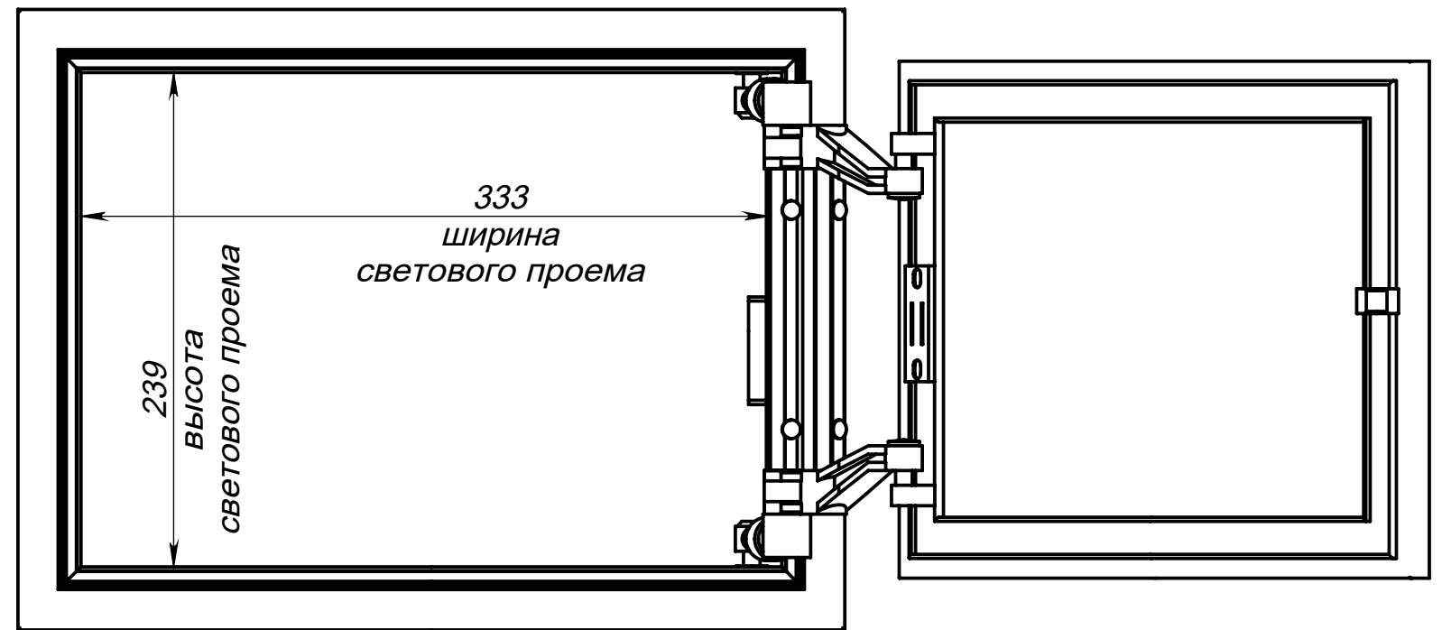
Вид спереди на люк (дверь открывается до 135 градусов)
