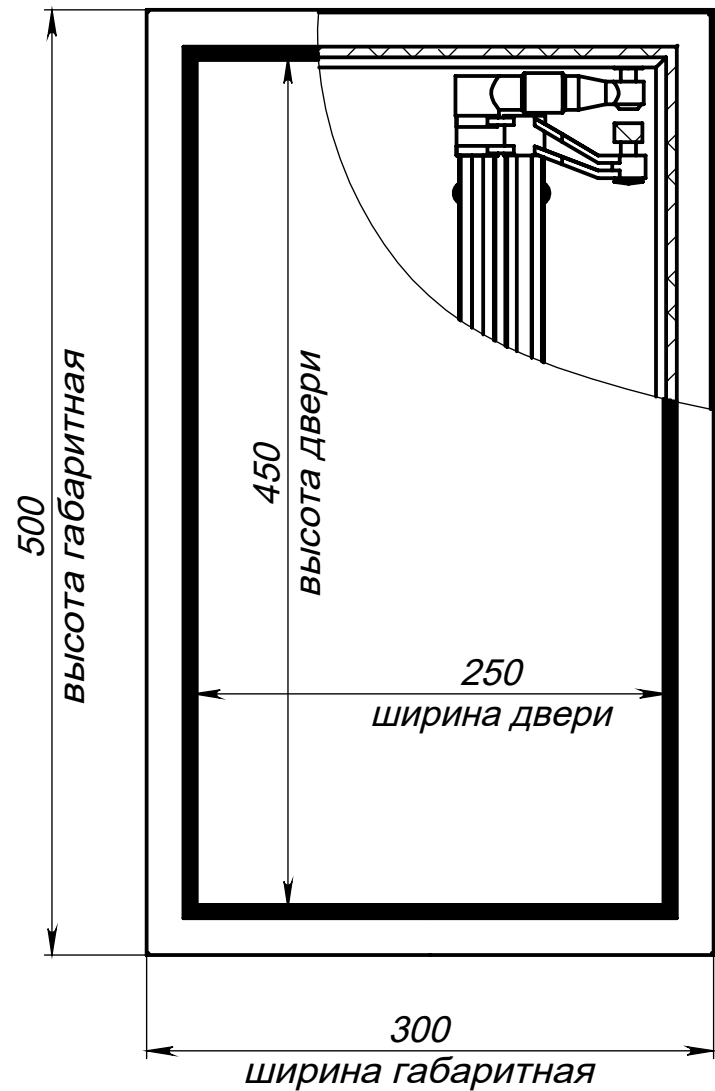
Вид спереди на люк (дверь закрыта)
