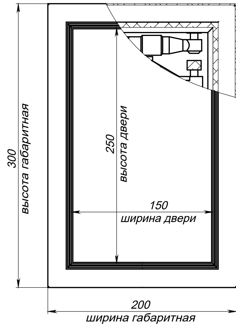
Вид сверху на люк - в разрезе (дверь закрыта)
