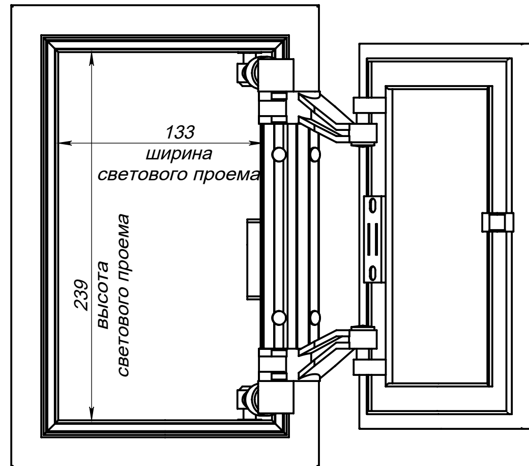
Вид спереди на люк (дверь открывается до 135 градусов)
