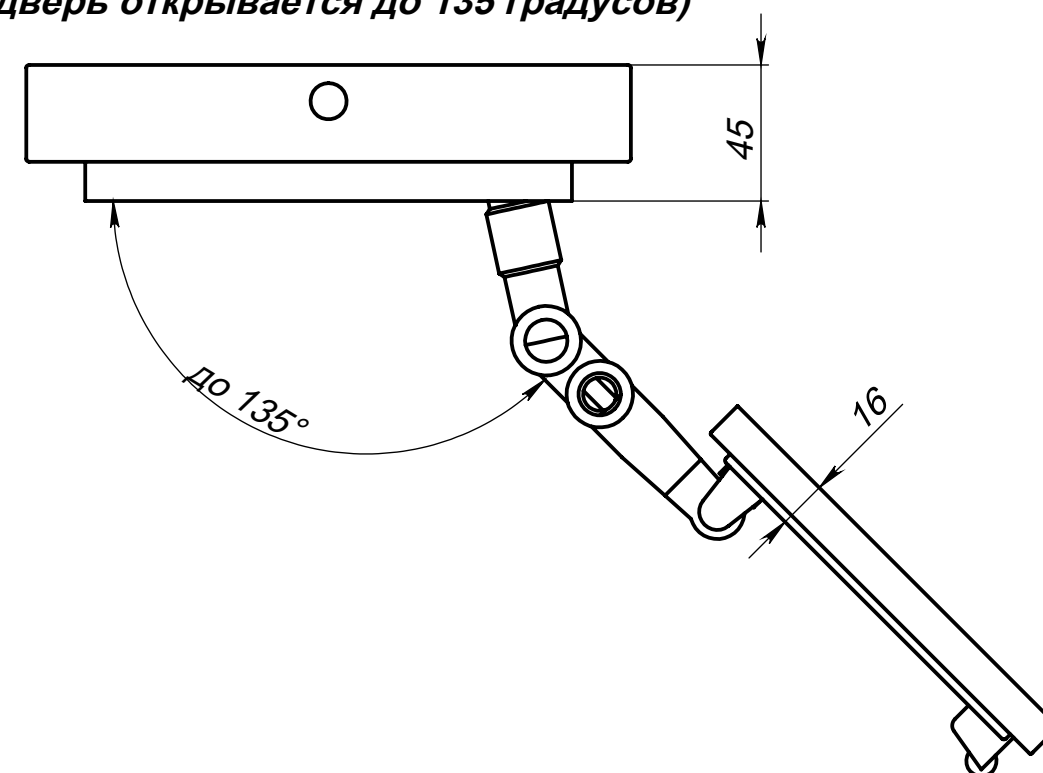
Вид сверху на люк (дверь открывается до 135 градусов)
