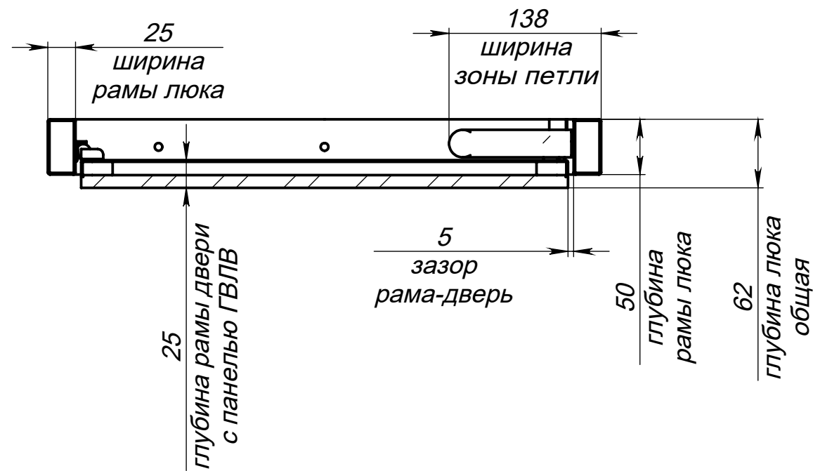
Вид сверху на люк - в разрезе (дверь закрыта)
