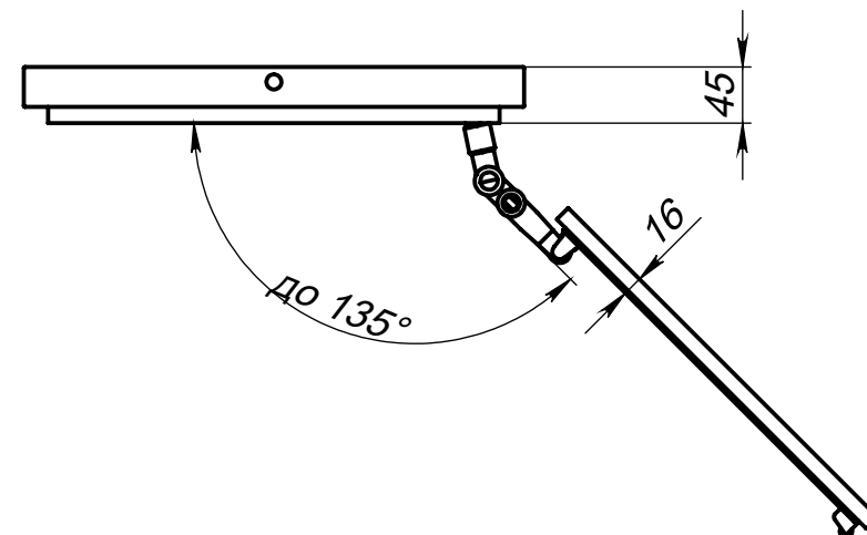
Вид сверху на люк (дверь открывается до 135 градусов)
