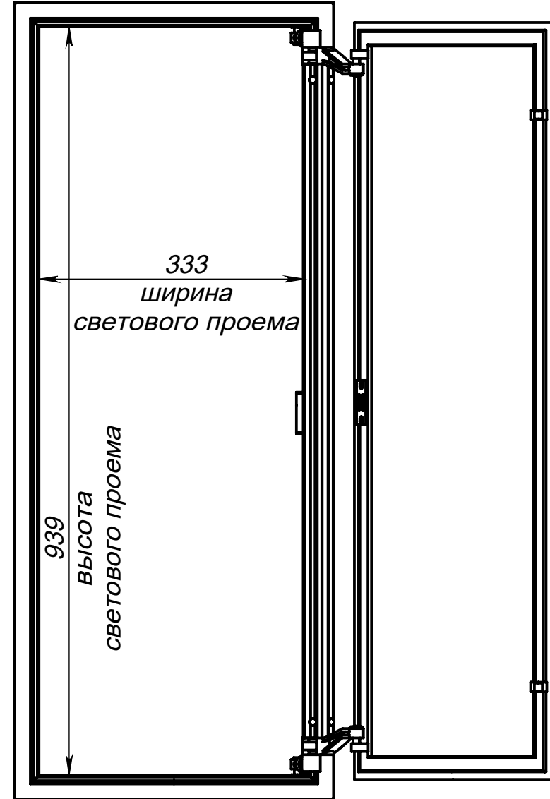
Вид спереди на люк (дверь открывается до 135 градусов)
