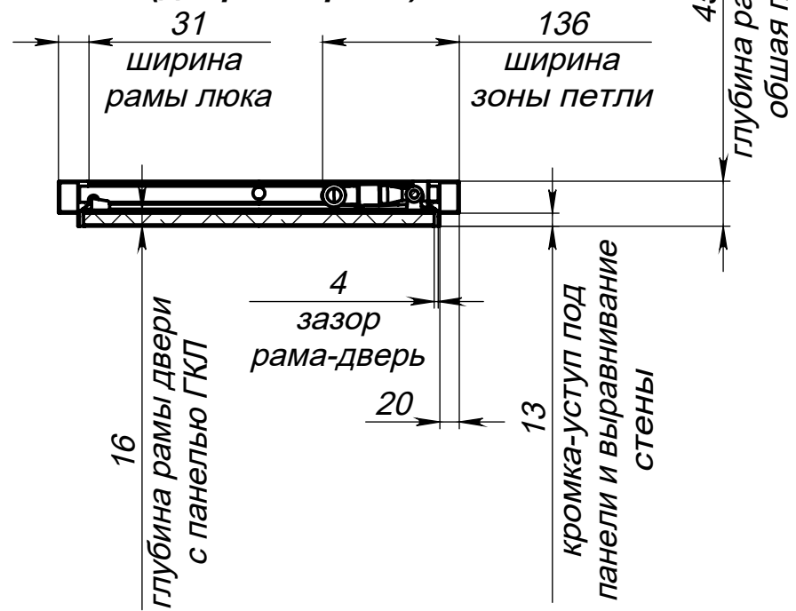
Вид сверху на люк - в разрезе (дверь закрыта)
