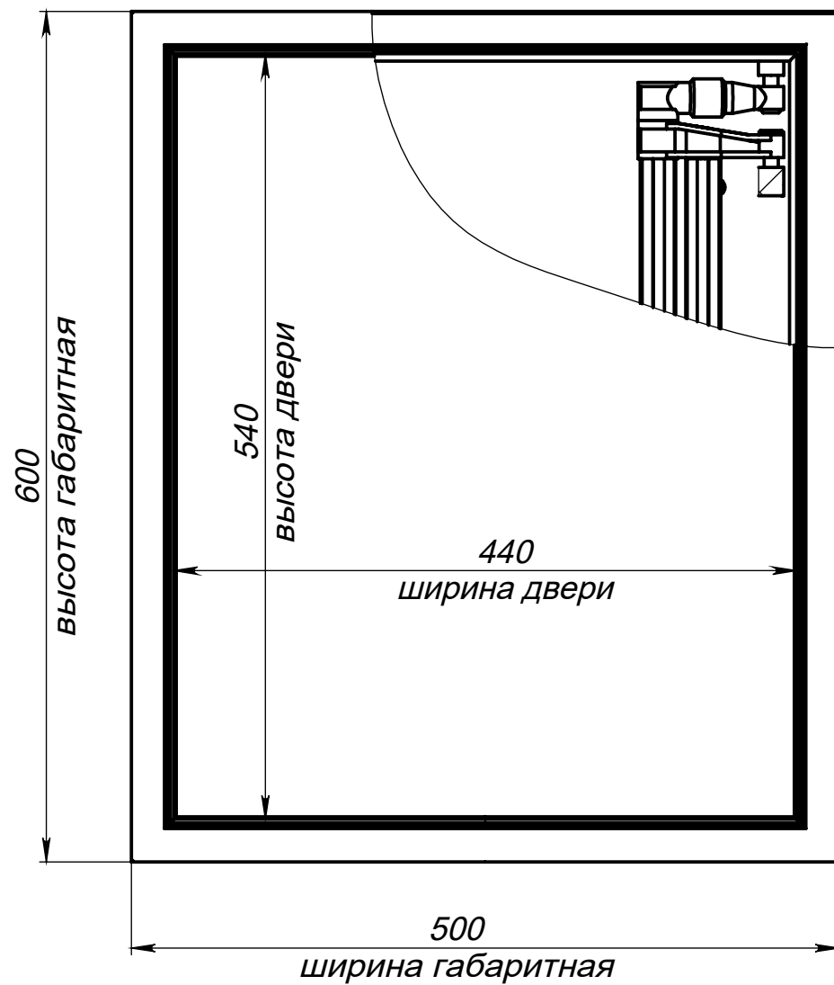
Вид спереди на люк (дверь закрыта)
