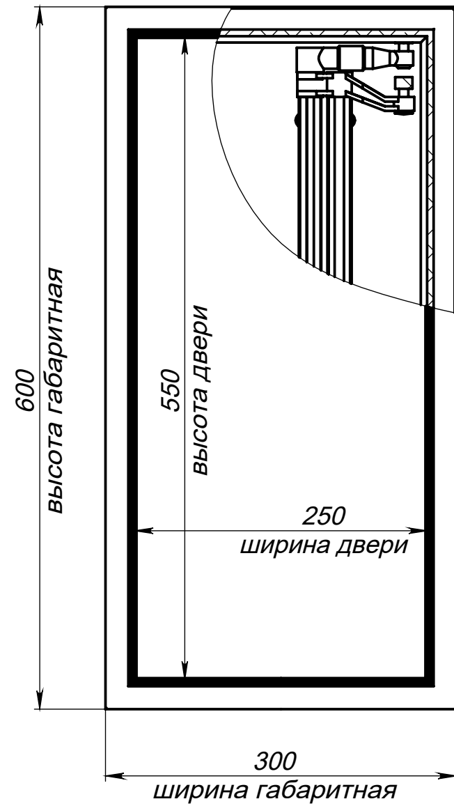
Вид спереди на люк (дверь закрыта)
