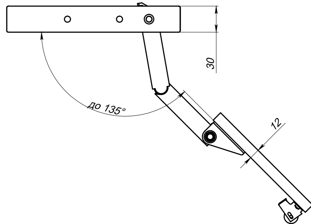
Вид сверху на люк (дверь открывается до 135 градусов)
