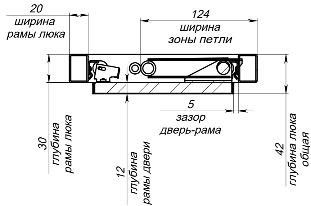
Вид сверху на люк - в разрезе (дверь закрыта)
