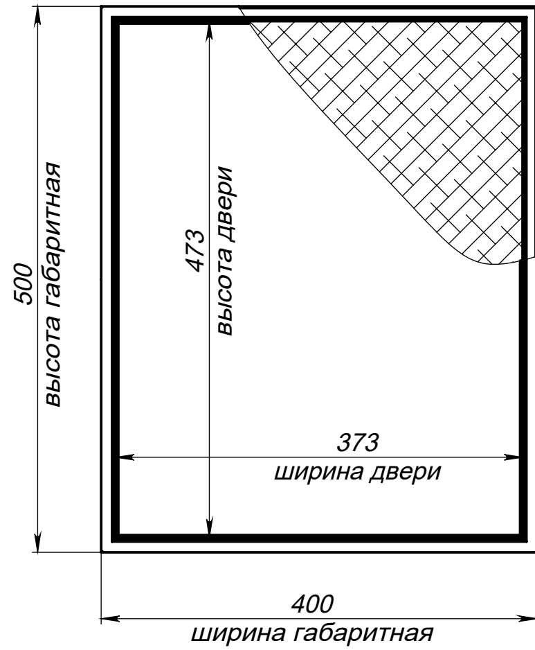
Вид спереди на люк (съемная дверь установлена)
