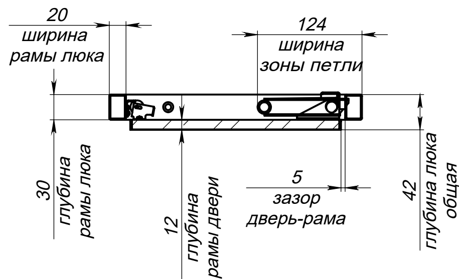
Вид сверху на люк - в разрезе (дверь закрыта)
