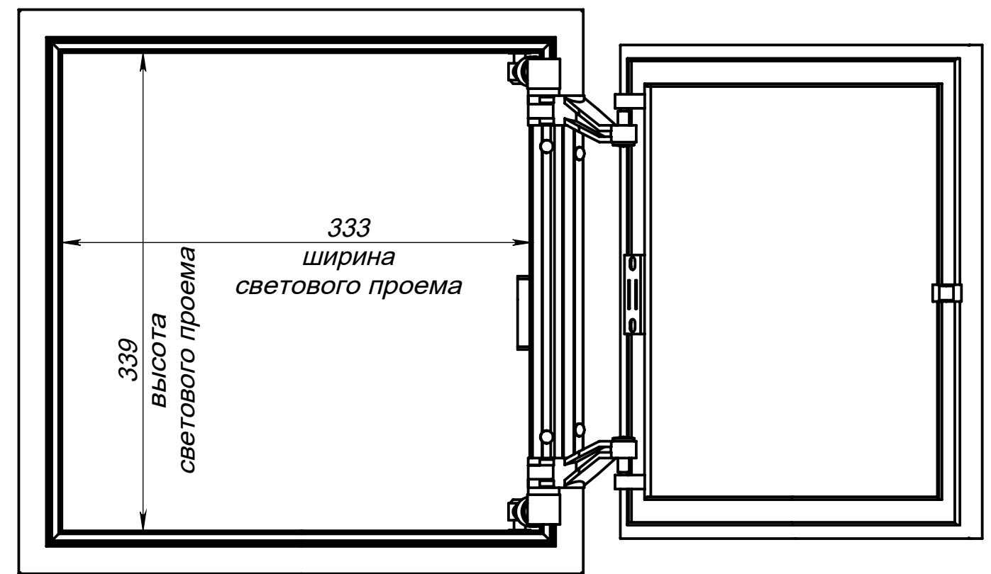
Вид спереди на люк (дверь открывается до 135 градусов)
