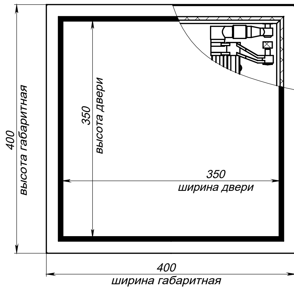
Вид спереди на люк (дверь закрыта)
