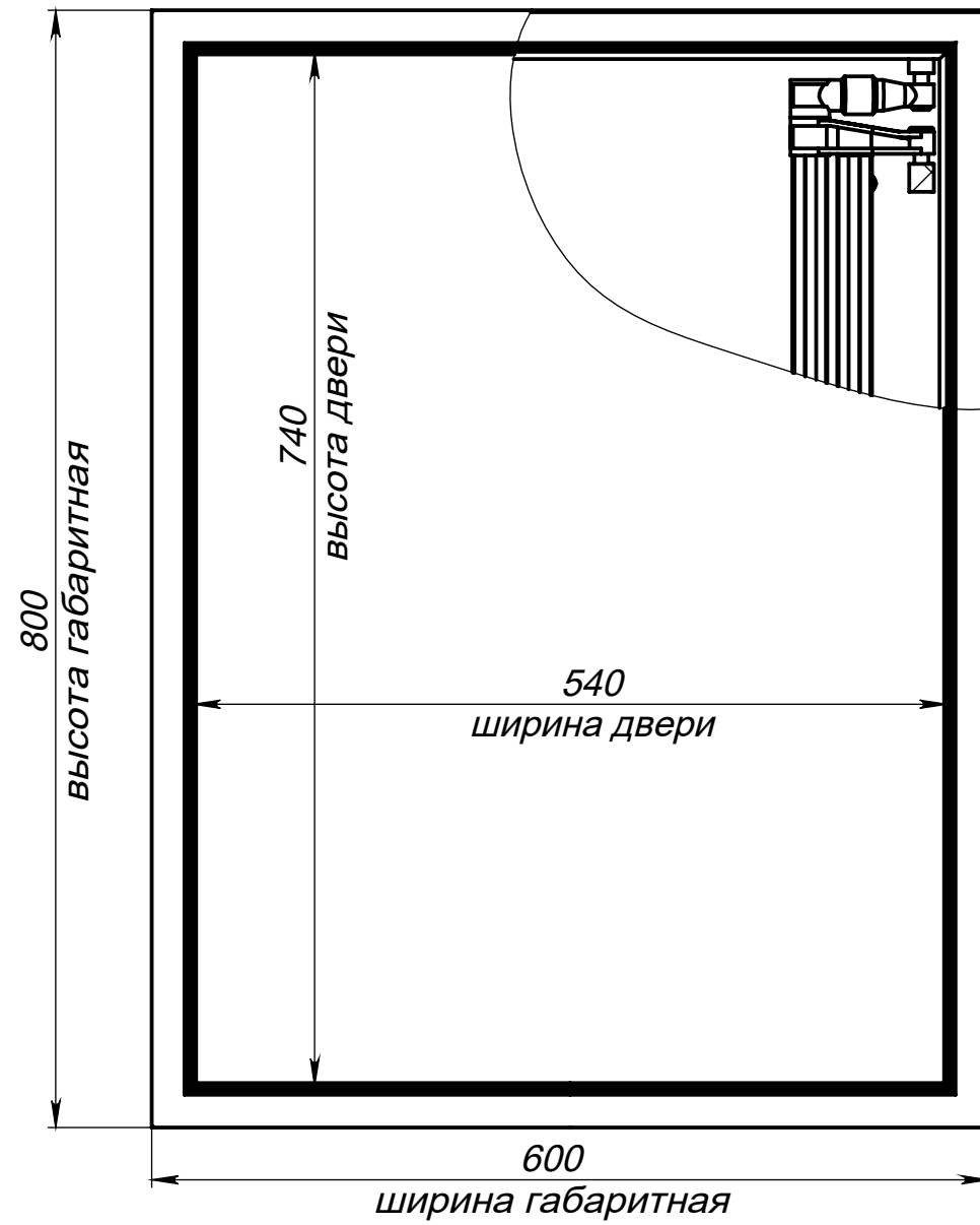
Вид спереди на люк (дверь закрыта)
