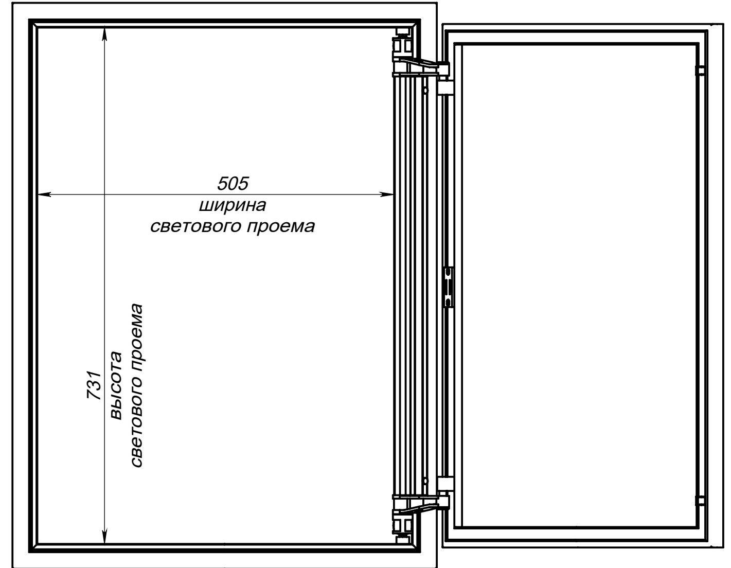
Вид спереди на люк (дверь открывается до 135 градусов)
