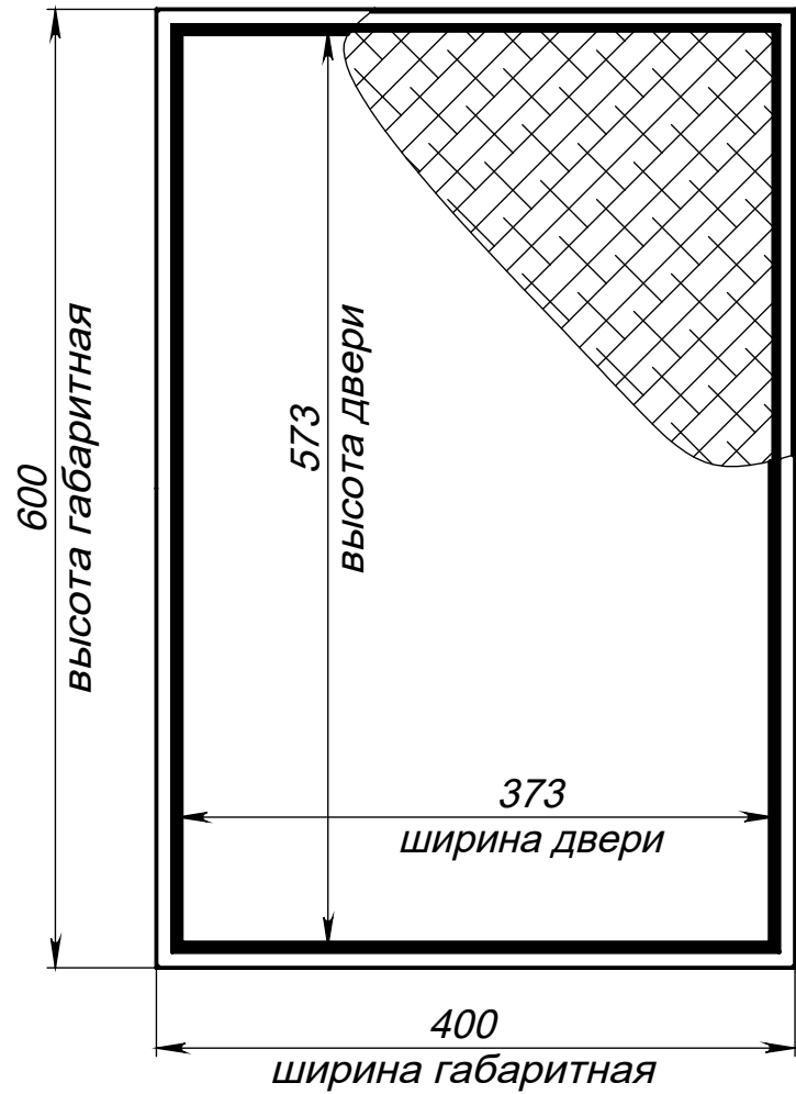
Вид спереди на люк (съемная дверь установлена)
