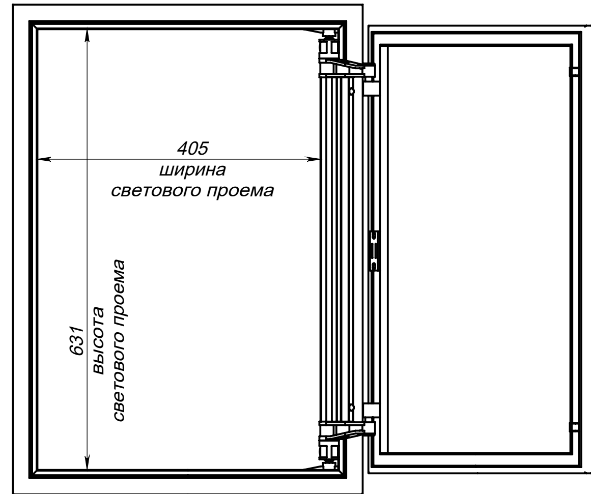
Вид спереди на люк (дверь открывается до 135 градусов)
