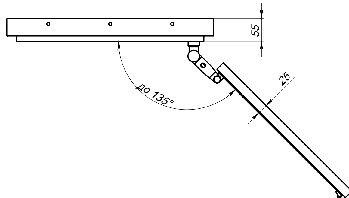
Вид сверху на люк (дверь открывается до 135 градусов)
