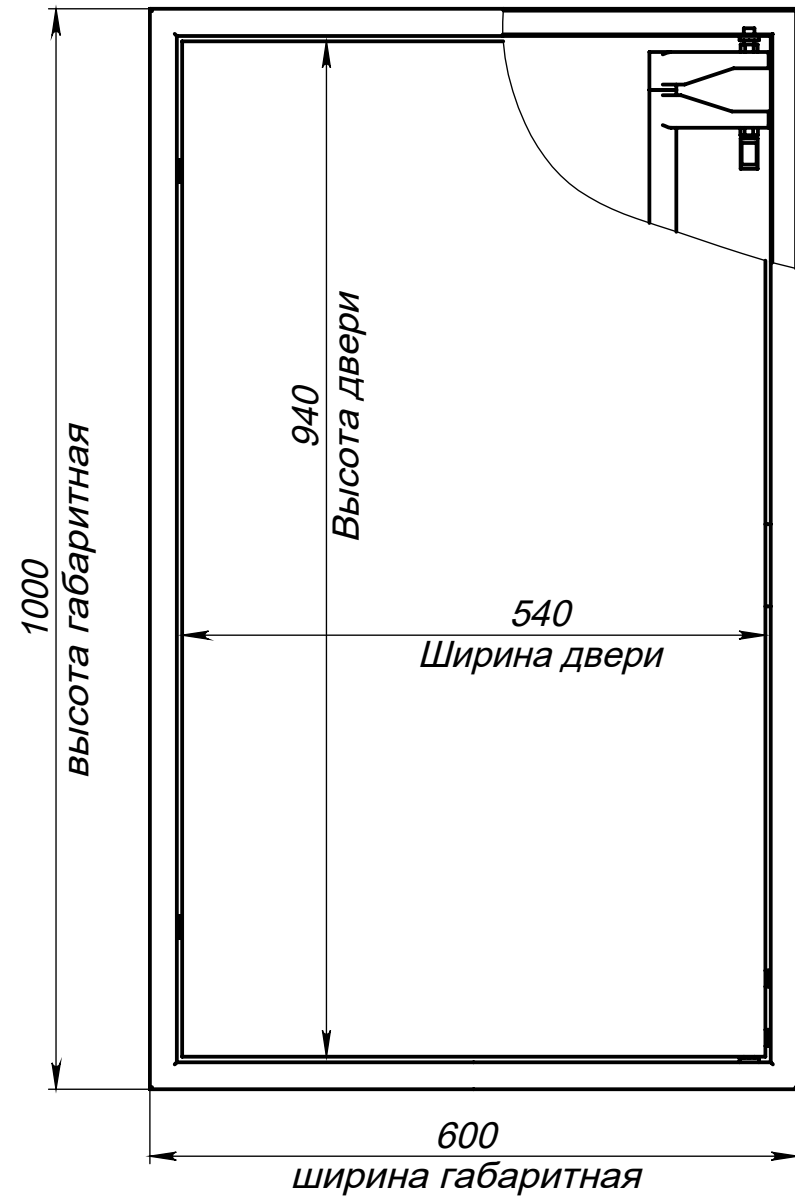
Вид сверху на люк - в разрезе (дверь закрыта)
