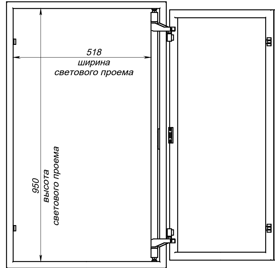
Вид спереди на люк (дверь открывается до 135 градусов)
