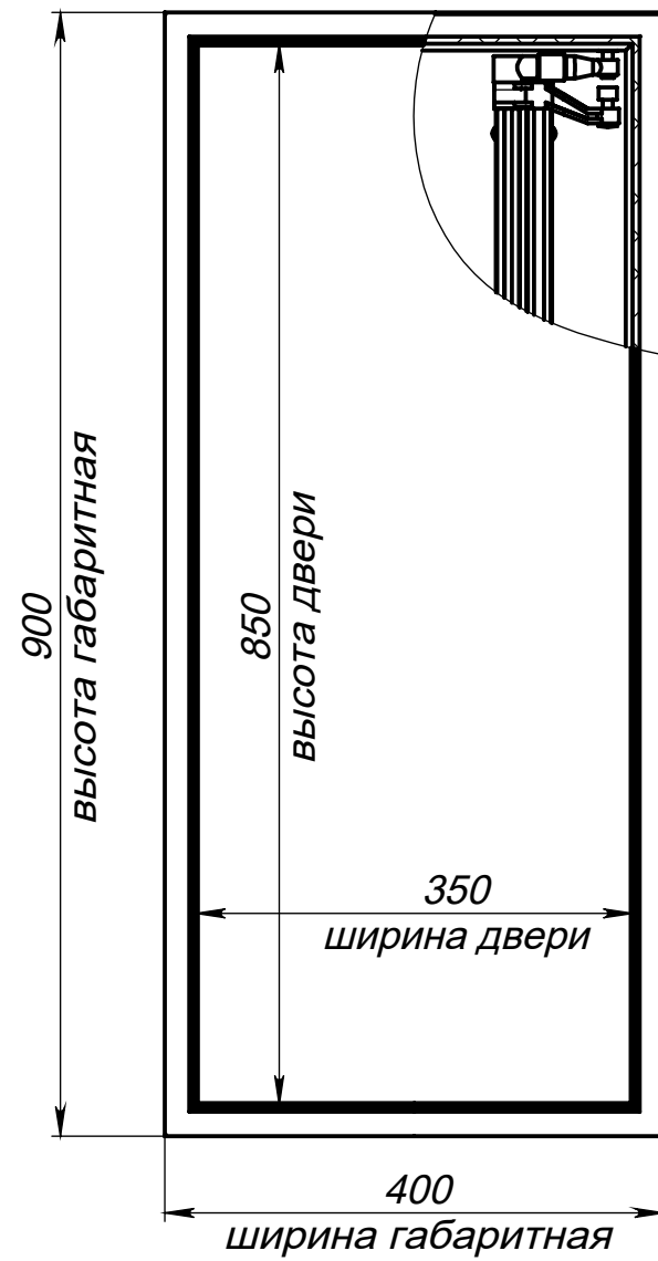
Вид спереди на люк (дверь закрыта)
