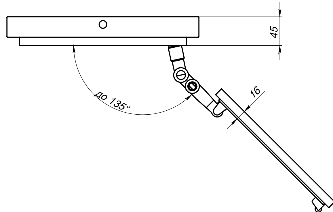
Вид сверху на люк (дверь открывается до 135 градусов)
