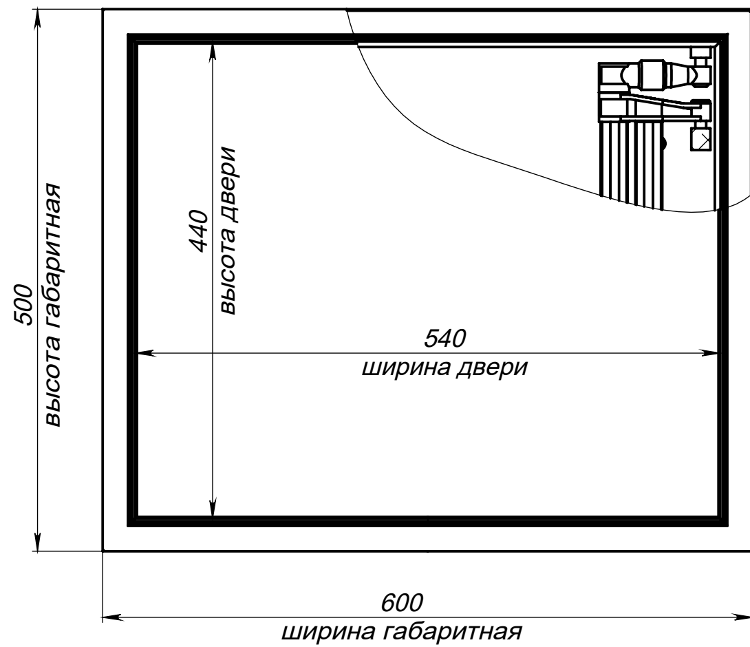
Вид сверху на люк - в разрезе (дверь закрыта)
