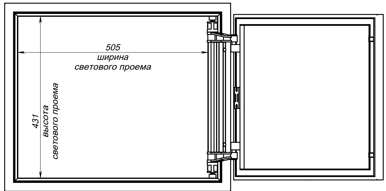
Вид спереди на люк (дверь открывается до 135 градусов)
