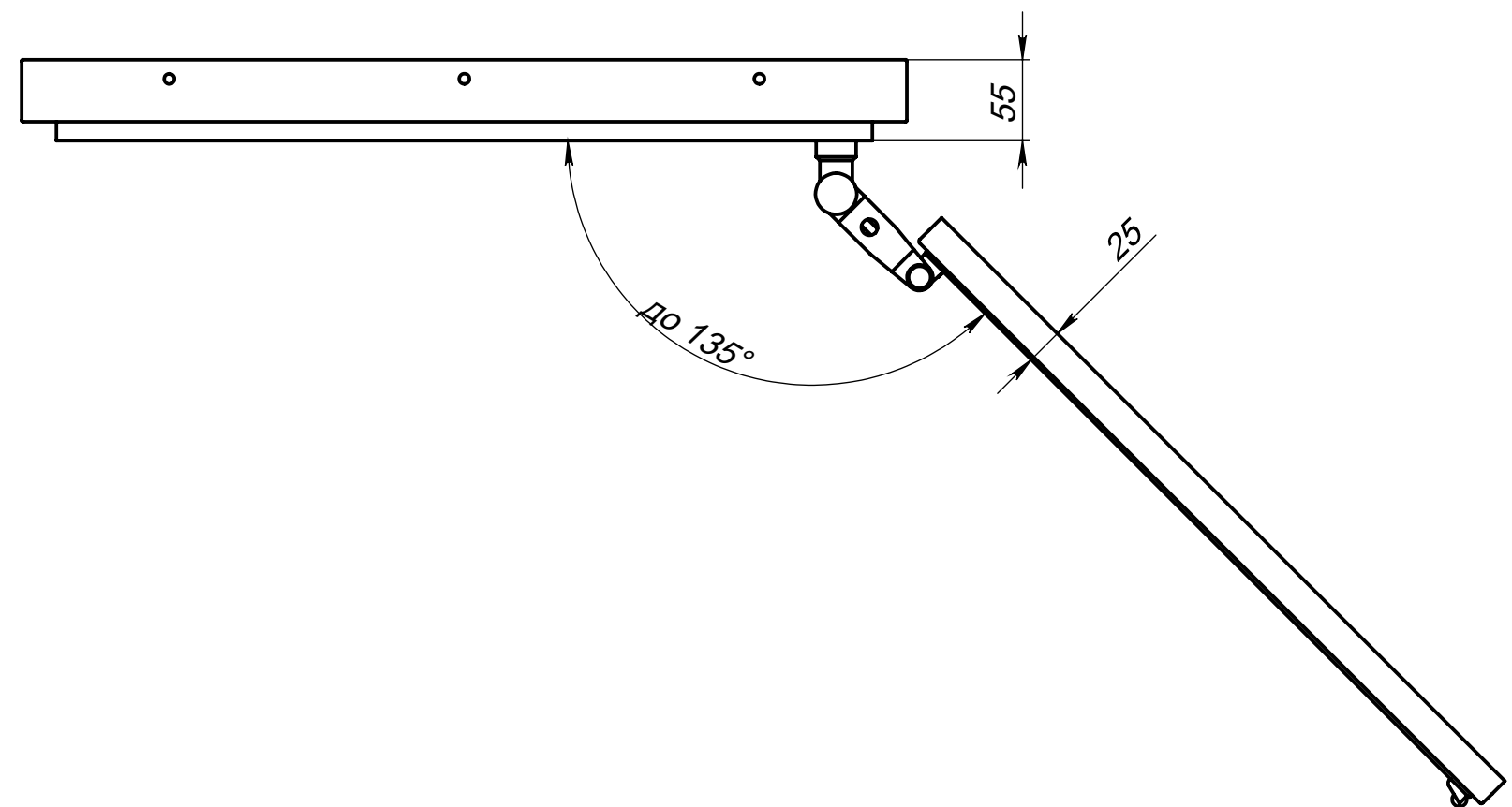
Вид сверху на люк (дверь открывается до 135 градусов)
