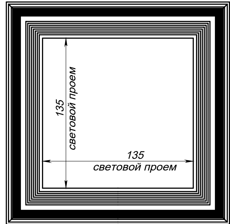
Вид сверху на люк (дверь не показана)
