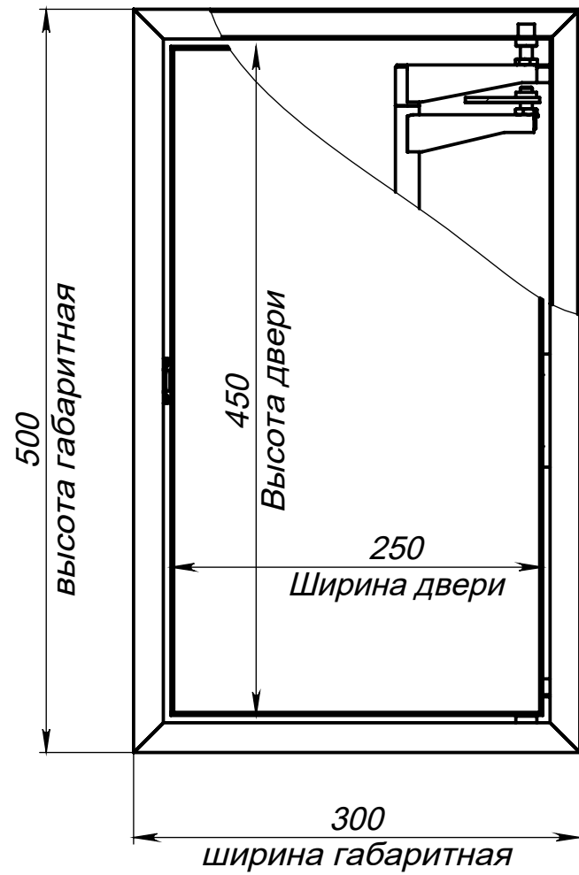
Вид спереди на люк (дверь закрыта)
