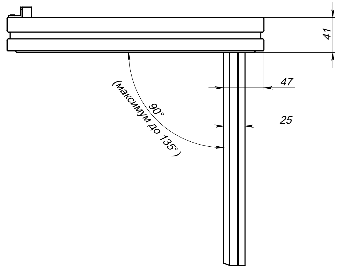
Вид сверху на люк (дверь открыта на 90 градусов)
