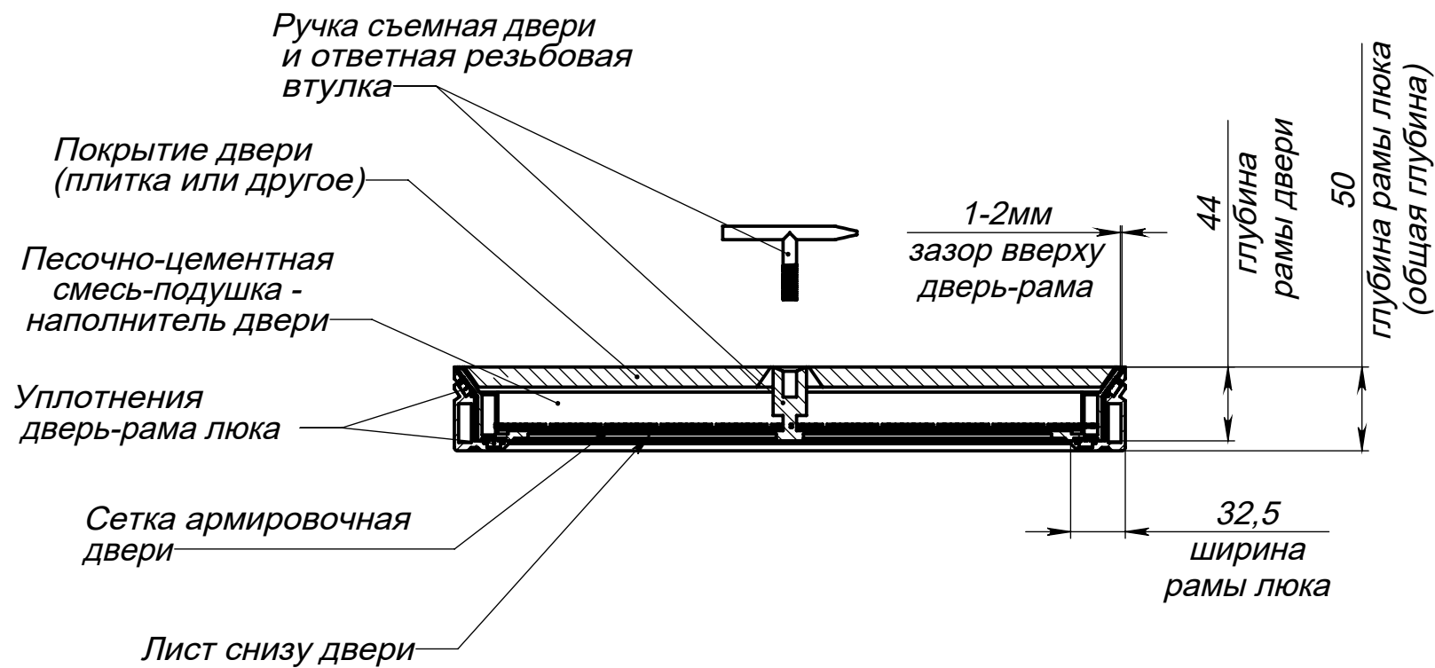
Вид сбоку на люк - в разрезе (дверь закрыта)
