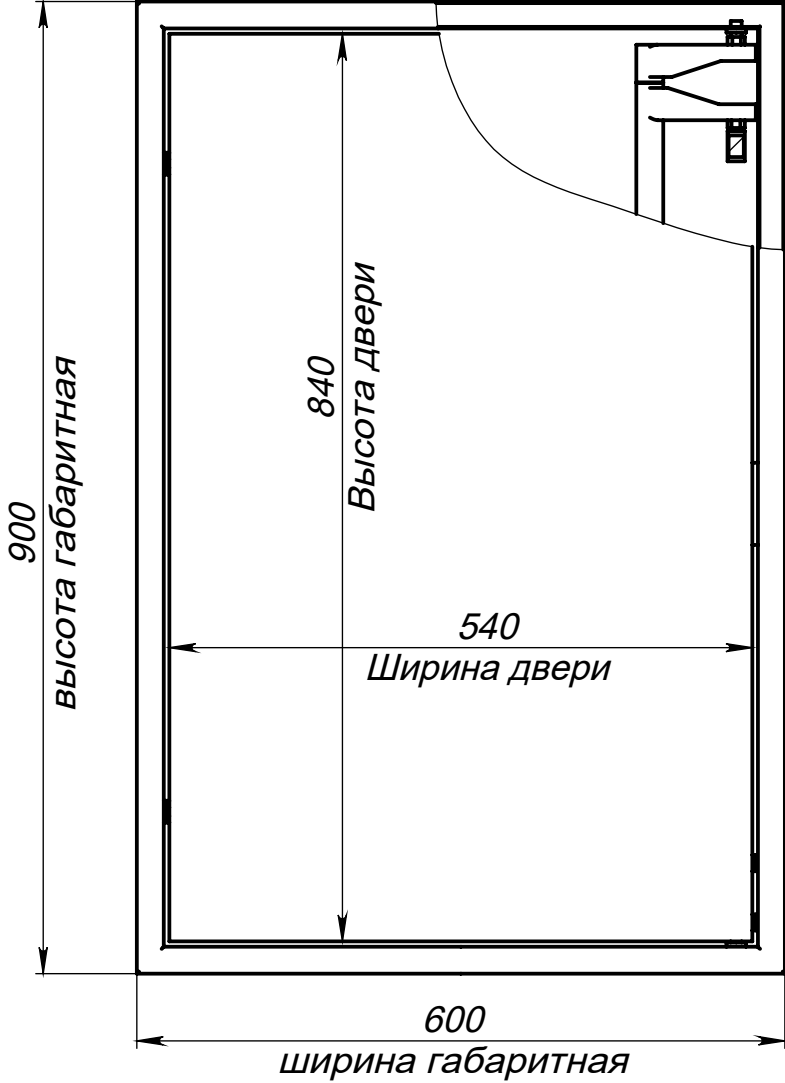
Вид спереди на люк (дверь закрыта)
