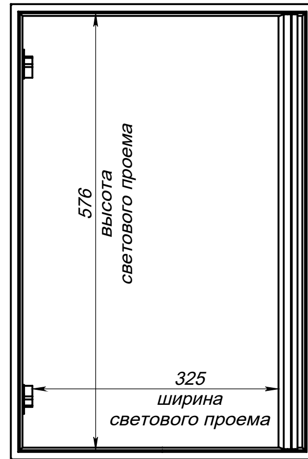
Вид спереди на люк (дверь открыта на 90 градусов)
