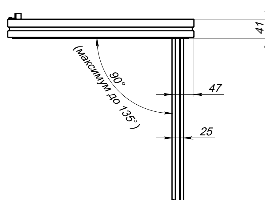
Вид сверху на люк (дверь открыта на 90 градусов)
