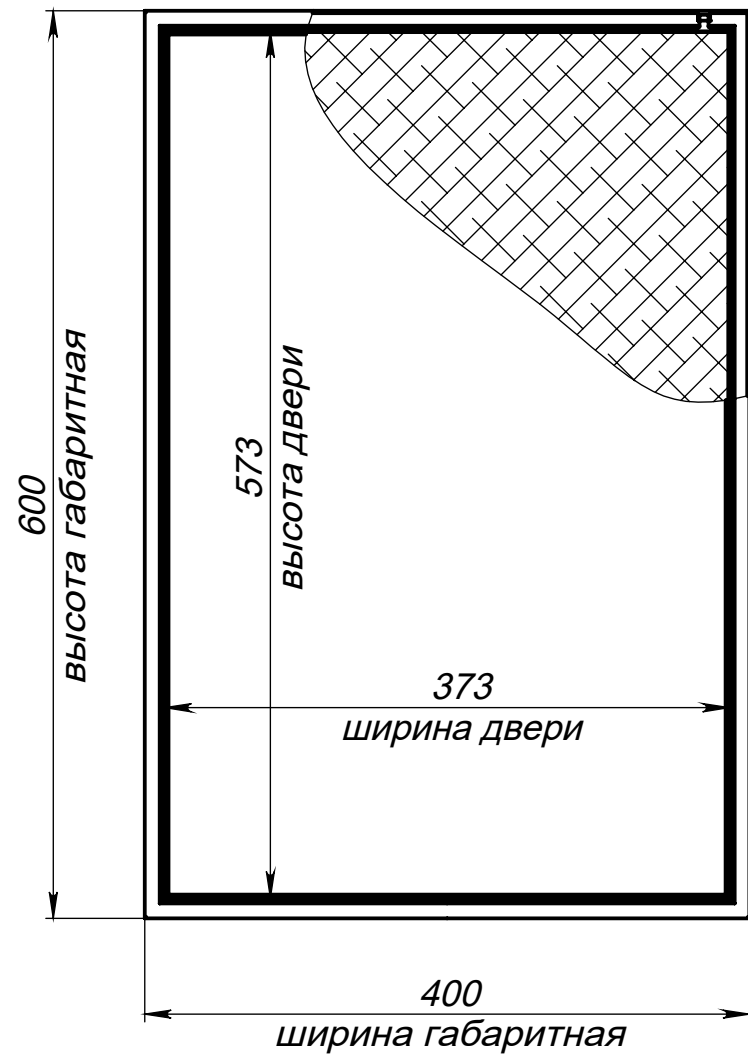
Вид спереди на люк (дверь закрыта)
