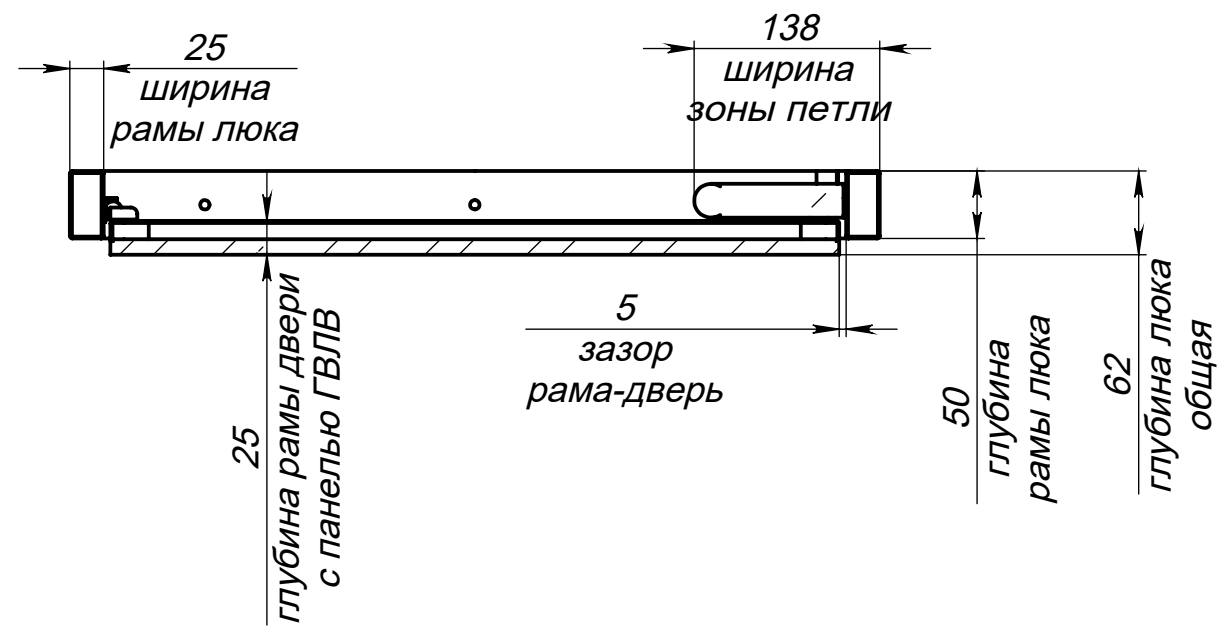
Вид сверху на люк - в разрезе (дверь закрыта)
