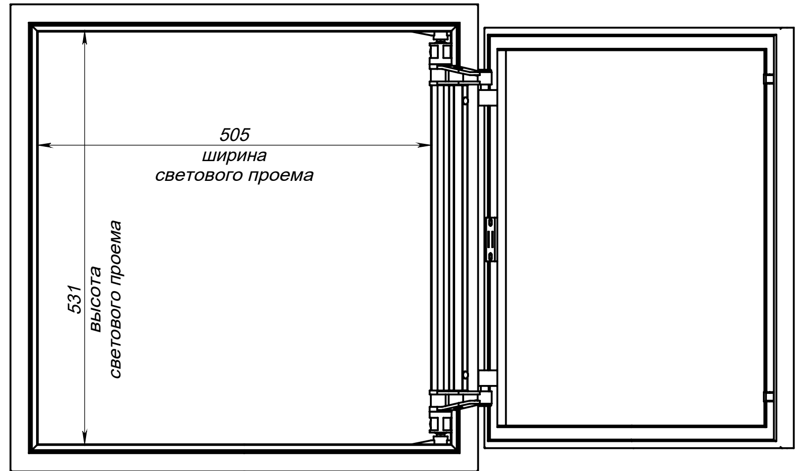
Вид спереди на люк (дверь открывается до 135 градусов)
