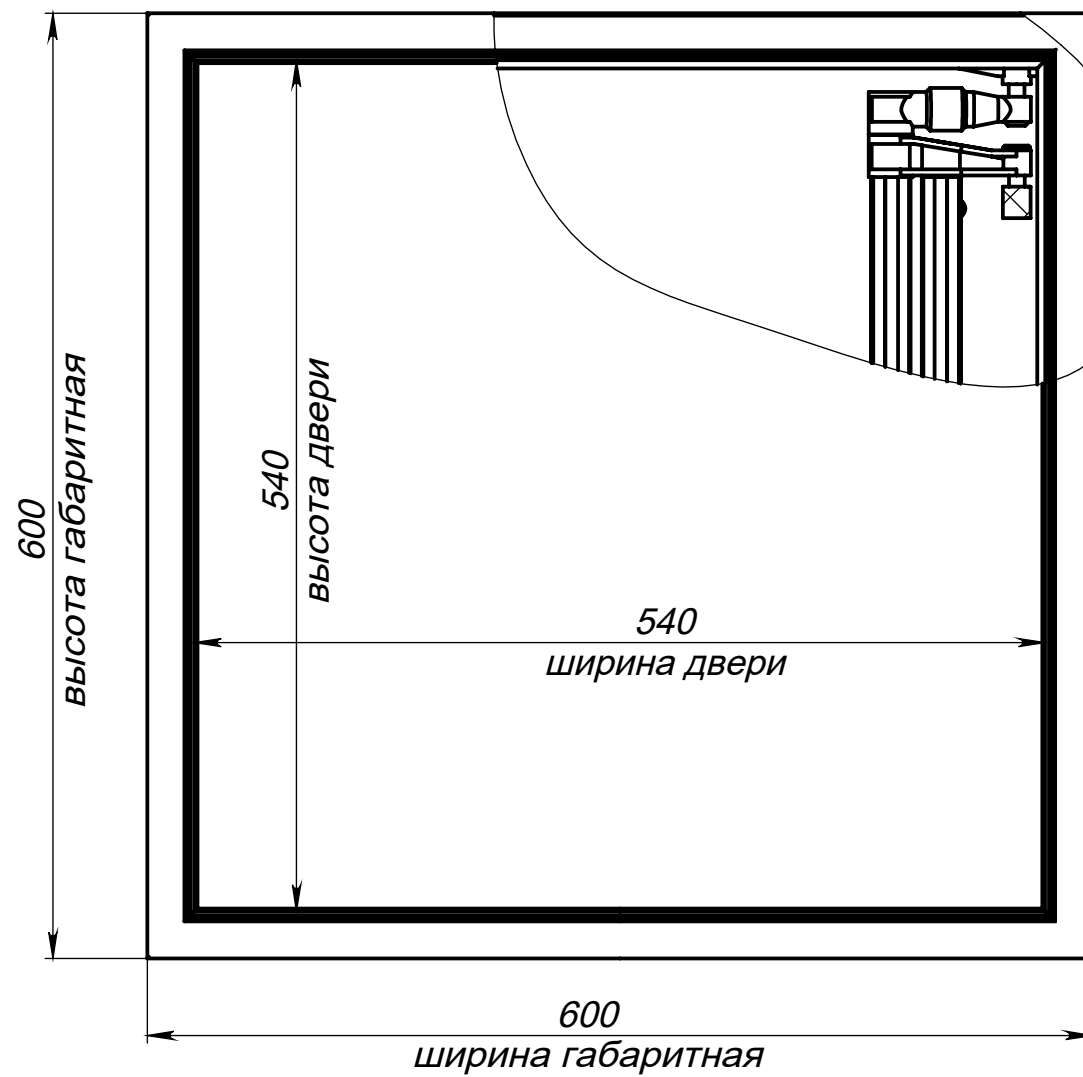
Вид спереди на люк (дверь закрыта)
