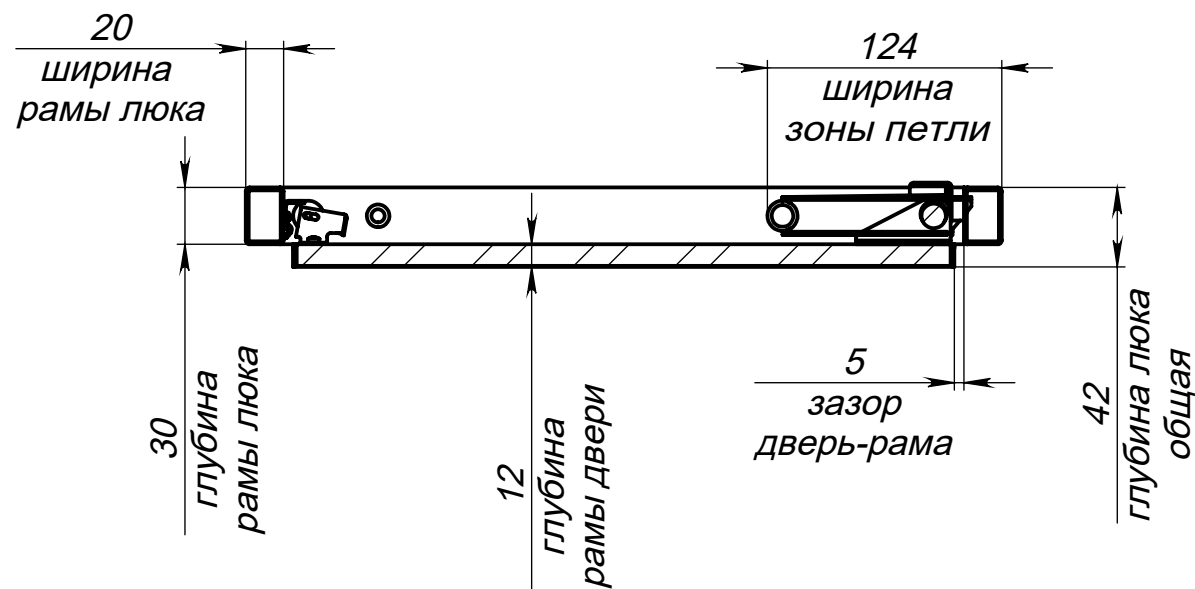
Вид сверху на люк - в разрезе (дверь закрыта)
