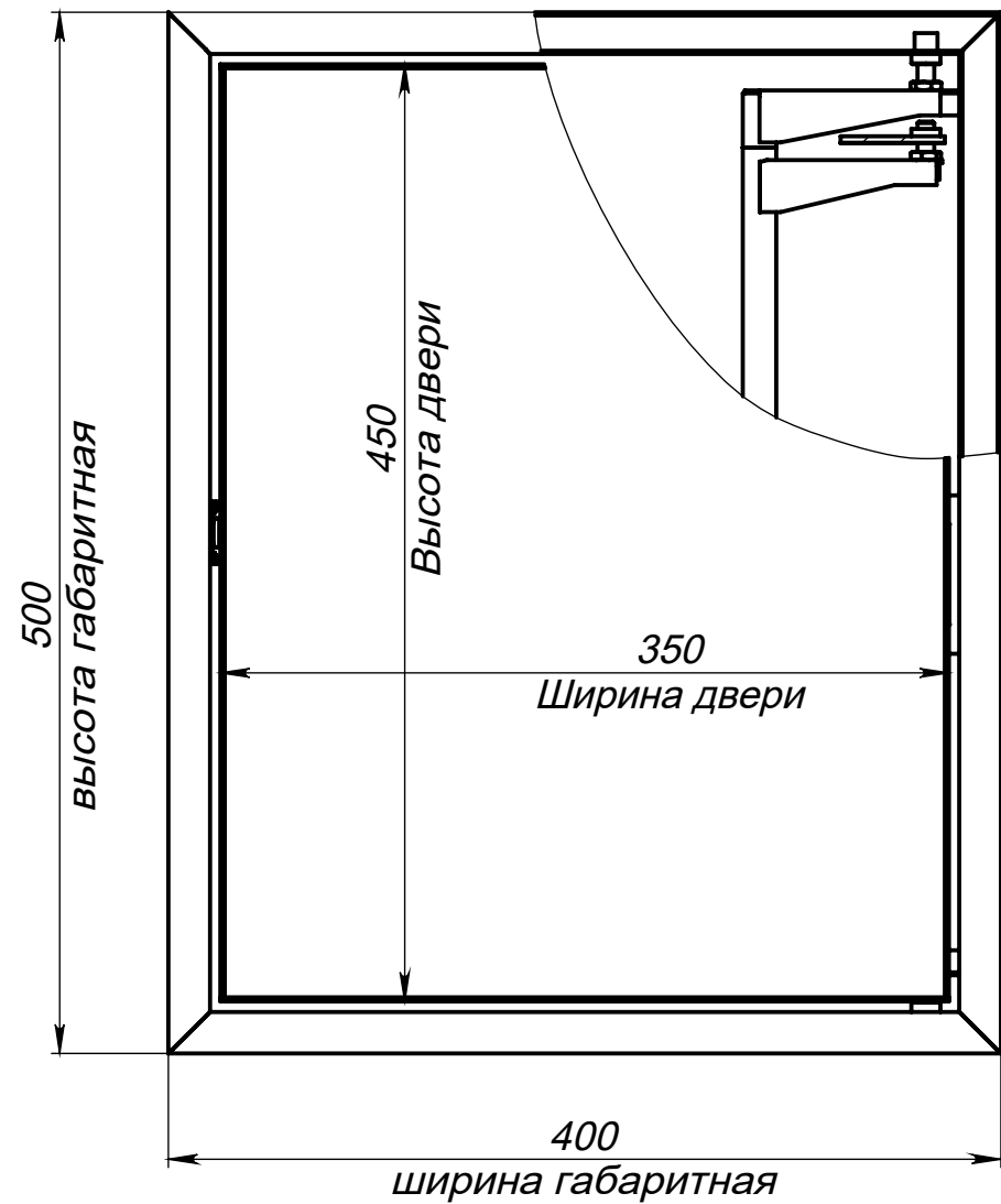
Вид спереди на люк (дверь закрыта)
