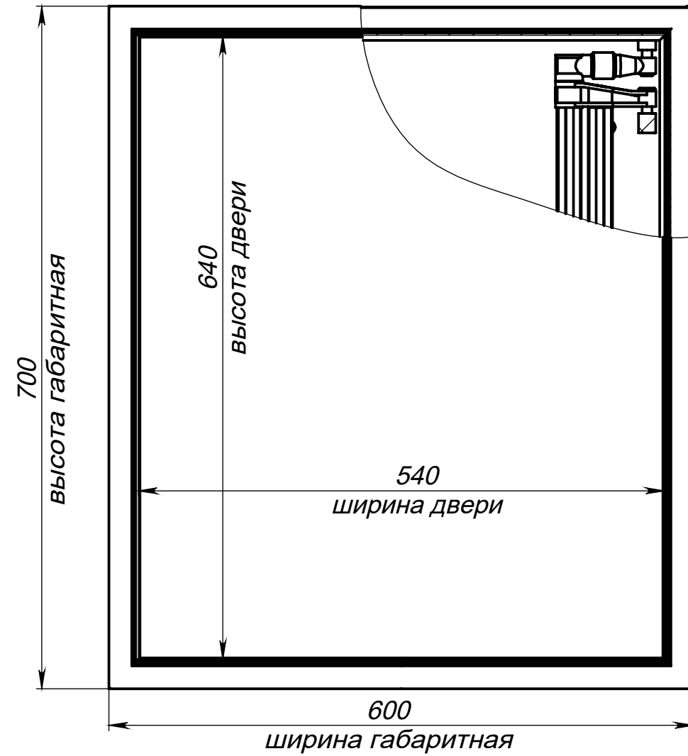
Вид сверху на люк - в разрезе (дверь закрыта)
